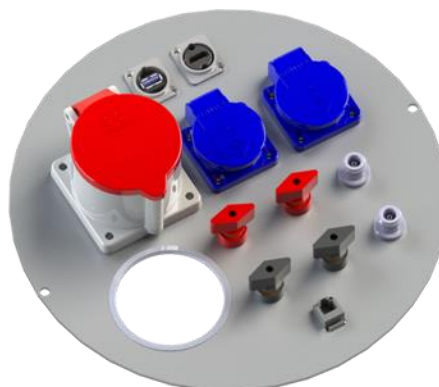
Beispiel für eine kundenspezifische Prüflingsversorgung
